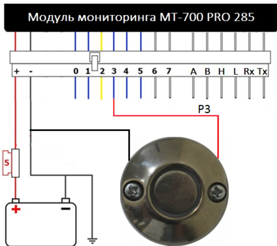
Рисунок 2 – Схема подключения iButton по 1-Wire к MT-700 Pro 285
